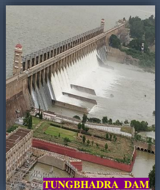
TUNGBHADRA DAM
